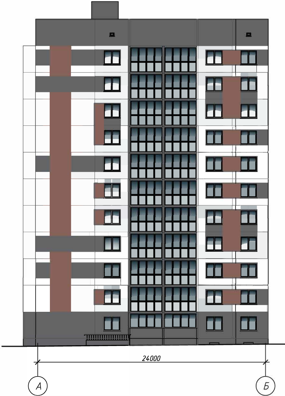
Фасад в осях А-Б
